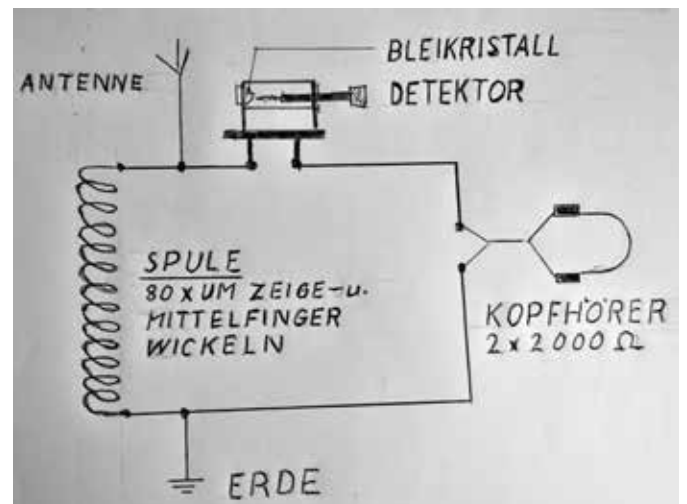
Das Verdrahtungsschema.
